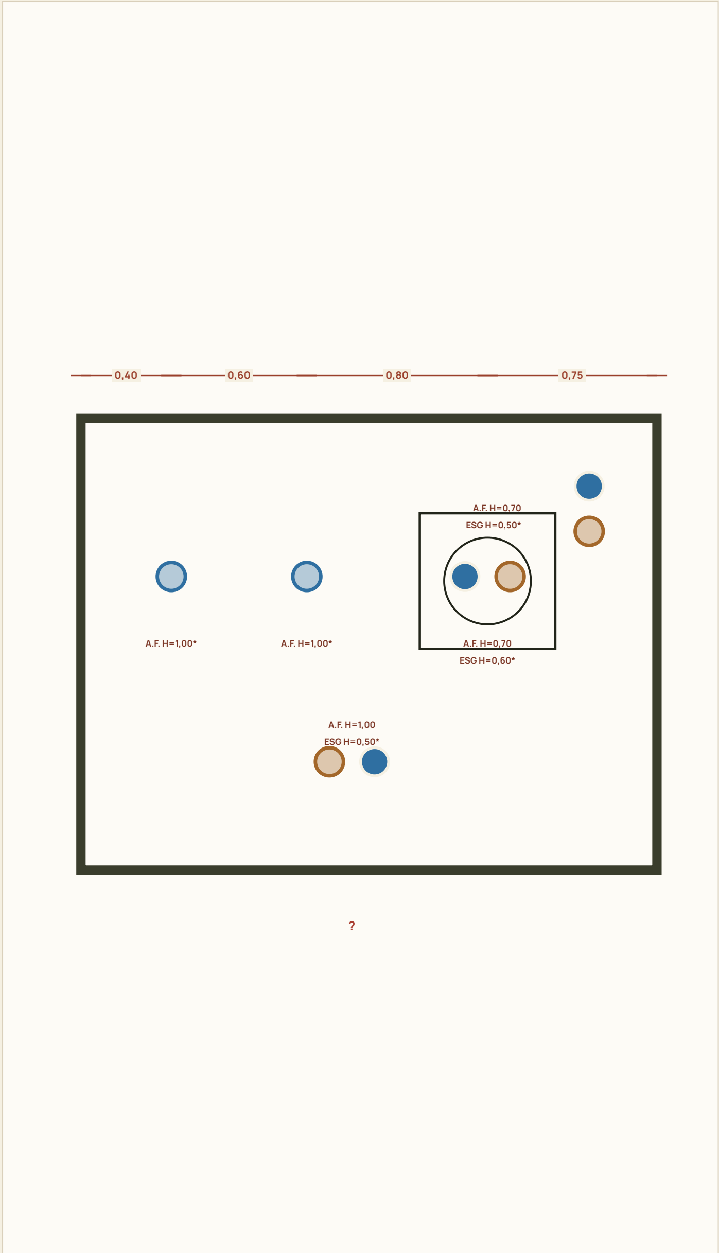
Lavanderia · planta de pontos hidráulicos ESCALA 1/17
